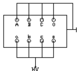
图 6-11 变压器接法
