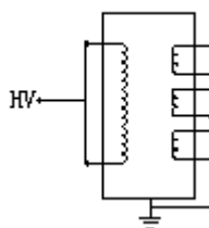
图 6-2 PT 接法
