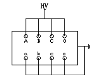
图 6-10 变压器接法
