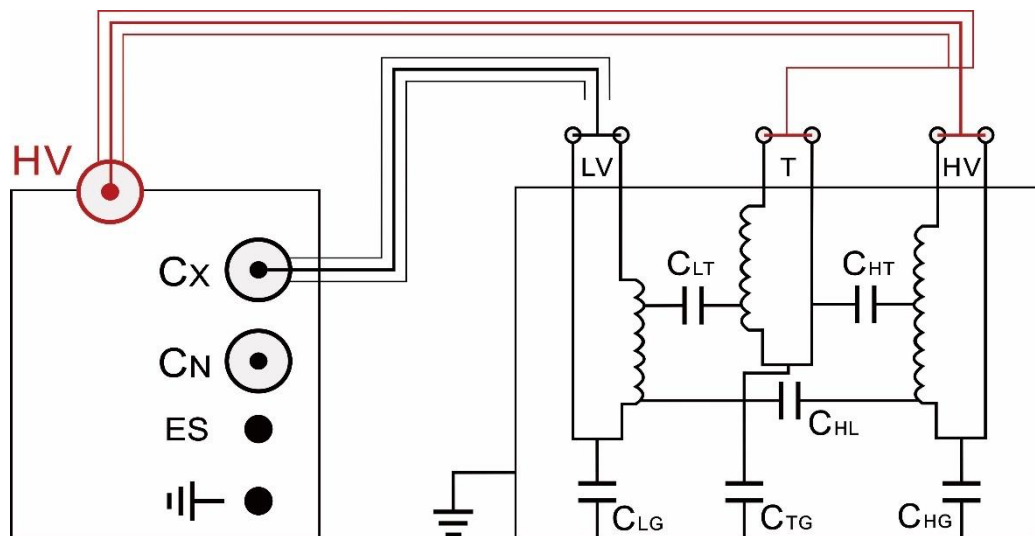
(4)、三绕组变压器 C_{LG}+C_{LT} 测试接线 (高压线屏蔽接 HV 绕组)
