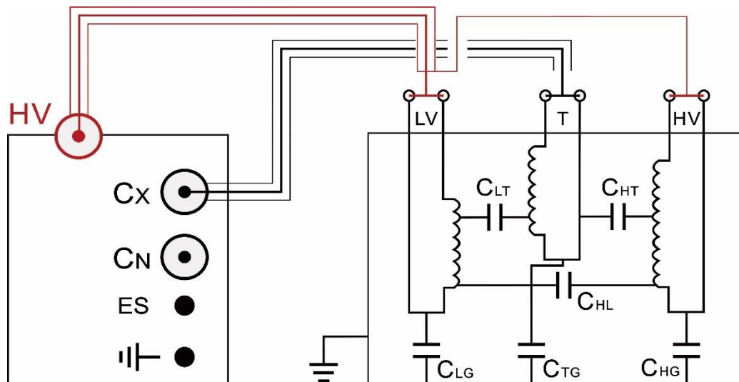
(5)、三绕组变压器 C_{TG}+C_{HT} 测试接线 (高压线屏蔽接 LV 绕组)
