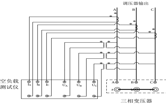
17) 使用 CT、PT 时单相变压器空载试验接线图
