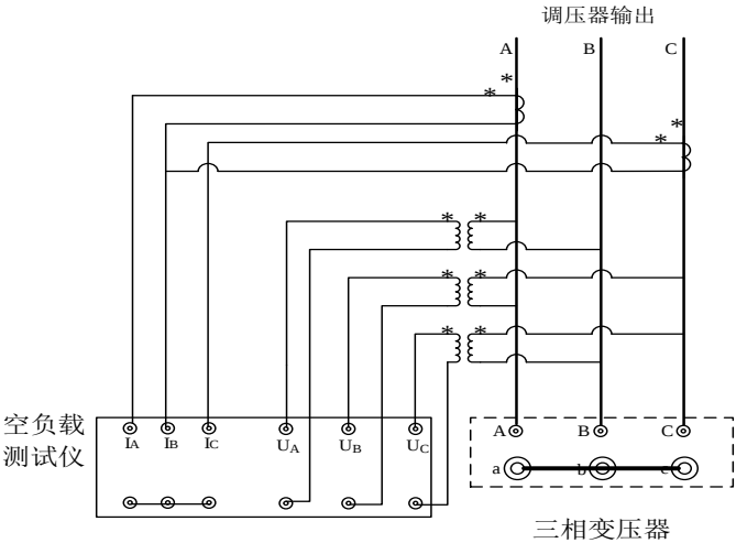
15) 使用 CT、PT 时三表法空载试验接线图
