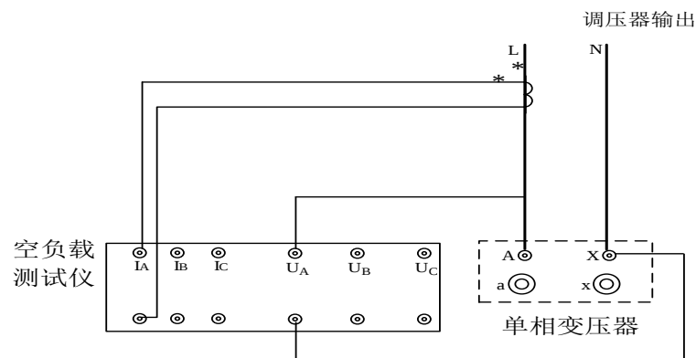
12) 使用 CT 时单相变压器负载试验接线图
