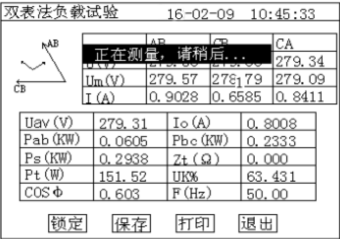
图 12 负载损耗正在测量计算页面
