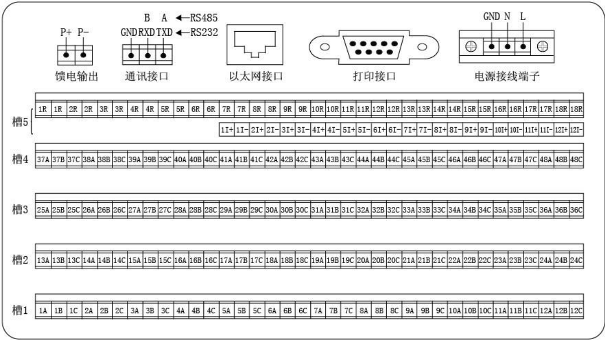
仪表尾部端子图
