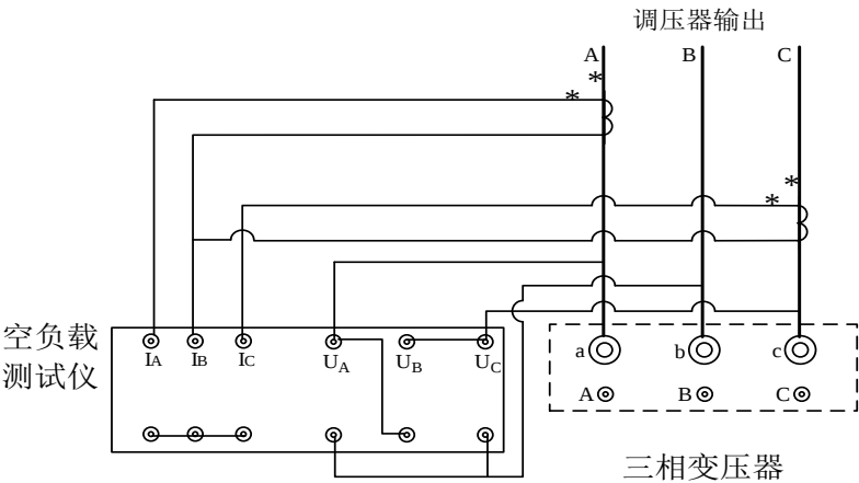
8) 使用 CT 时双表法负载试验接线图
