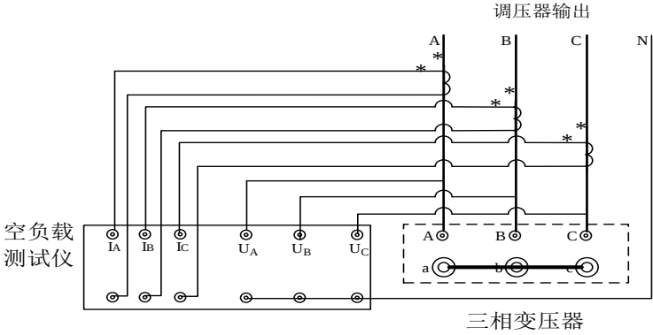
11) 使用 CT 时单相变压器空载试验接线图
