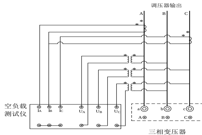
14) 使用 CT、PT 时双表法负载试验接线图
