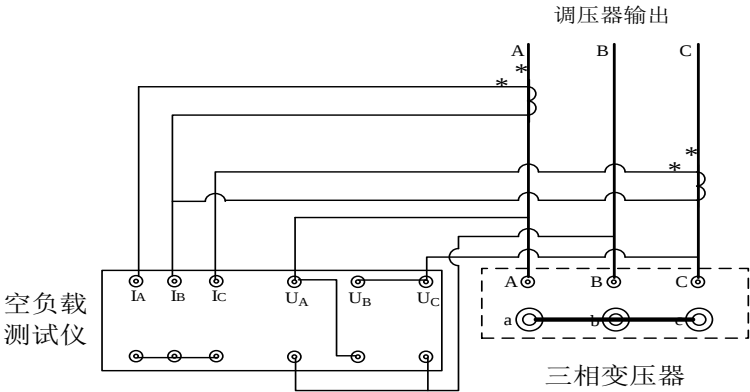
9) 使用 CT 时三表法空载试验接线图
