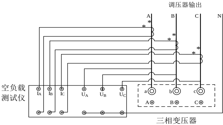
9) 使用 CT 时三表法空载试验接线图
