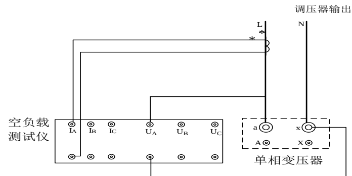
12) 使用 CT 时单相变压器负载试验接线图
