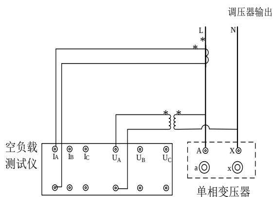
18) 使用 CT、PT 时单相变压器负载试验接线图
