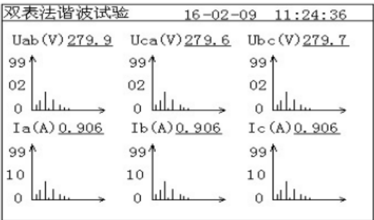
图 15 谐波分量频谱图页面
