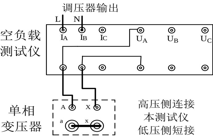
7) 使用 CT 时双表法空载试验接线图
