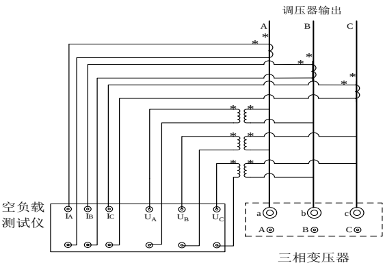
15) 使用 CT、PT 时三表法空载试验接线图
