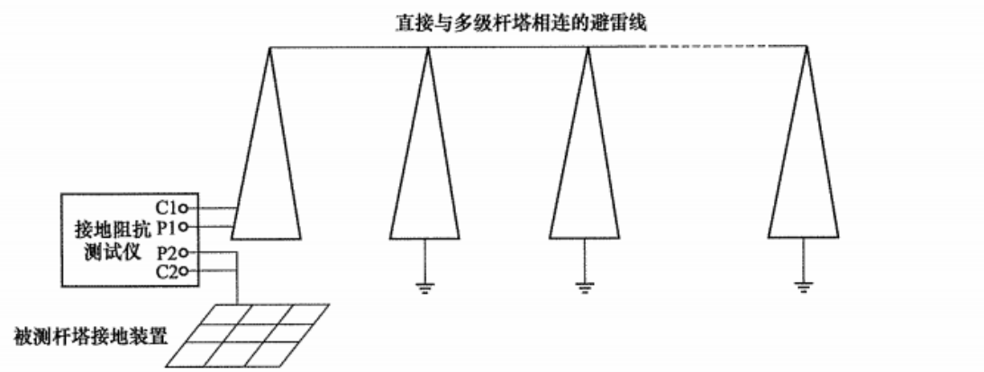
图 8 回路阻抗法测试杆塔接地阻抗示意图
