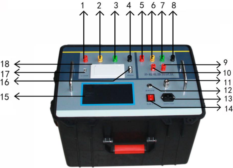
图 2 面板示意图
